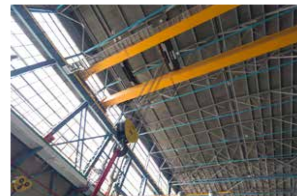
Кран грузоподъемностью 100/20т (заказчик РУП «Гродноэнерго»)
